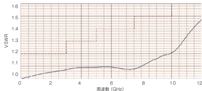
PCS3216 VSWR
