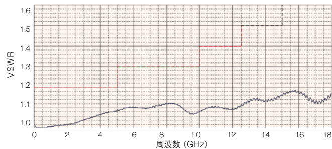
PCS1608 VSWR
