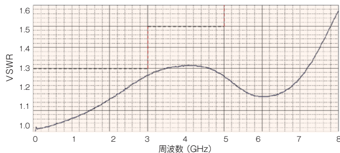
PCS6432 VSWR
