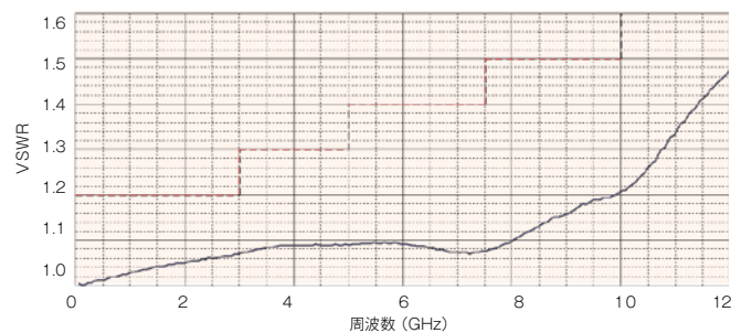
PCS3216 VSWR
