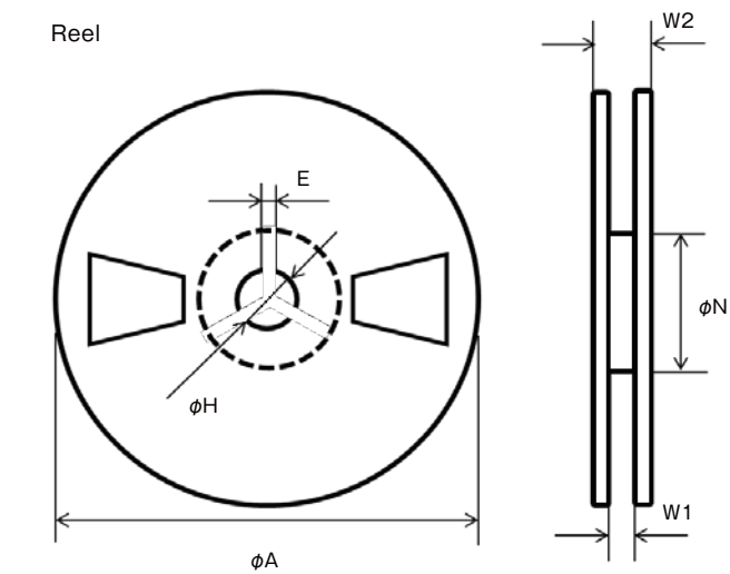
リールのサイズ
