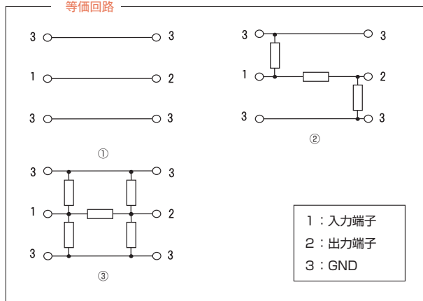
等価回路
