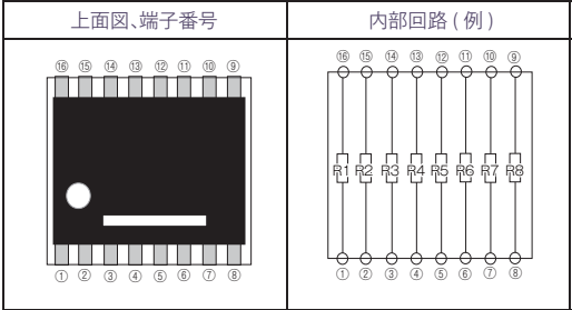
RM10280(10.2mm×7.2mm)
