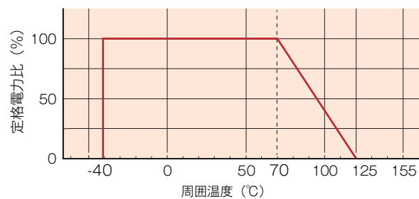
○ PAV3137S
