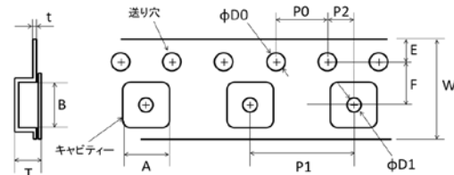
図-3 エンボステープ 8mm ピッチ
