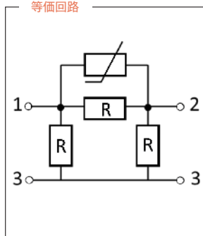
等価回路
