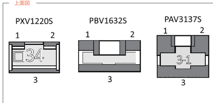
上面図
