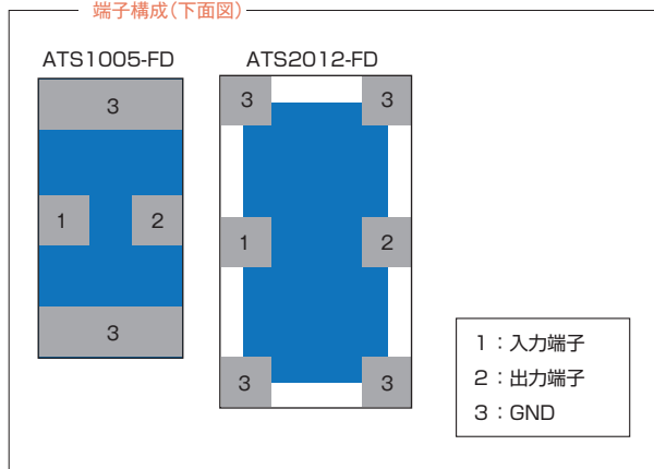
端子構成(下面図)
