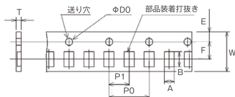
図-3 エンボステープ 8mm ピッチ
