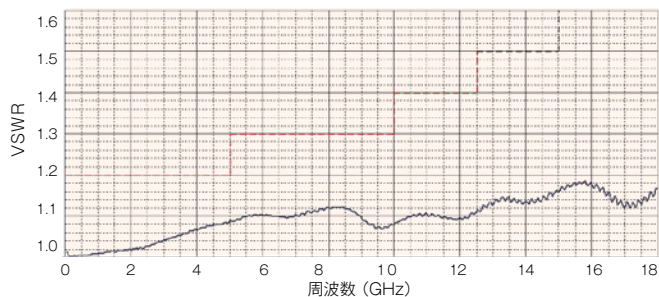
PCS1608 VSWR
