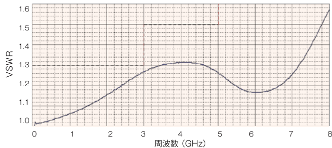
PCS6432 VSWR
