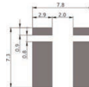
ランドパターン
