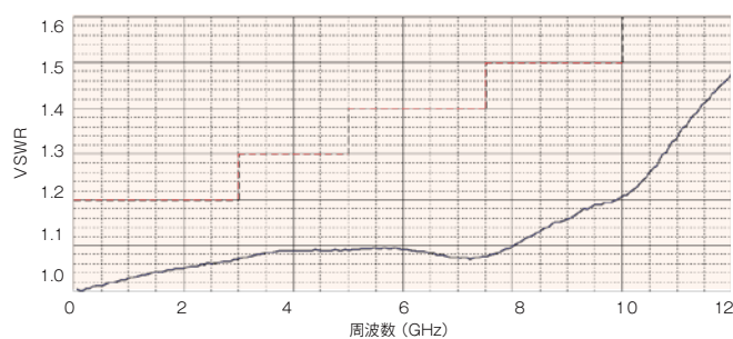
PCS3216 VSWR
