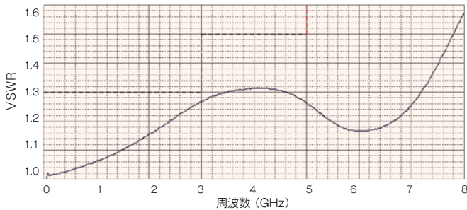
PCS6432 VSWR
