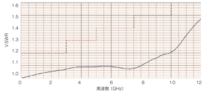
PCS3216 VSWR
