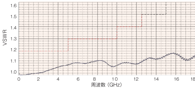
PCS1608 VSWR
